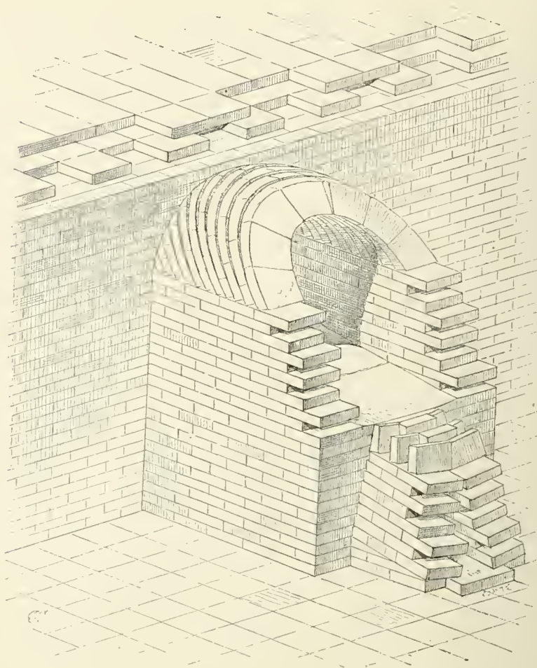
93. — Canal de Khorsabad, à voûte en plein cintre, d'après le géométral de Place, t. III, pl. 39, coupe CD.
